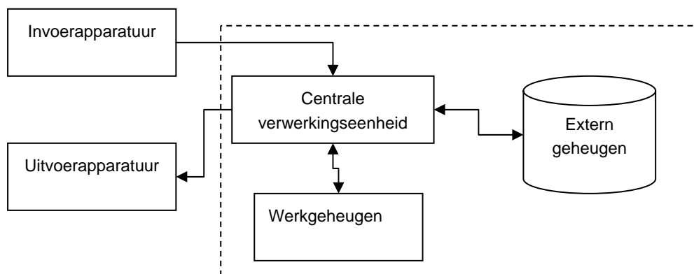
Figuur 1: basisarchitectuur van een computer ten behoeve van deze eindterm (Von Neumann architectuur)
